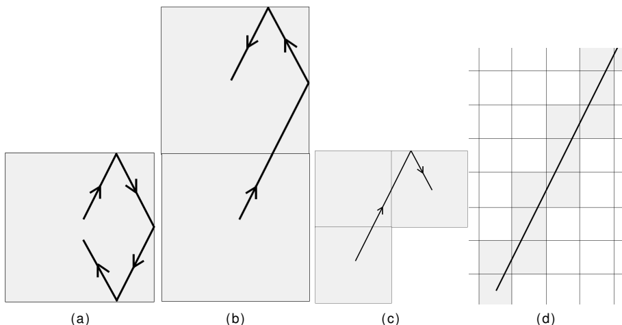
Abbildung 2: Aufklappen des Billardtisches.
