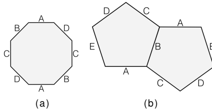
Abbildung 7: Ein Achteck oder zwei Fünfecke kann man zum Torus mit zwei Löchern zusammenkleben.
