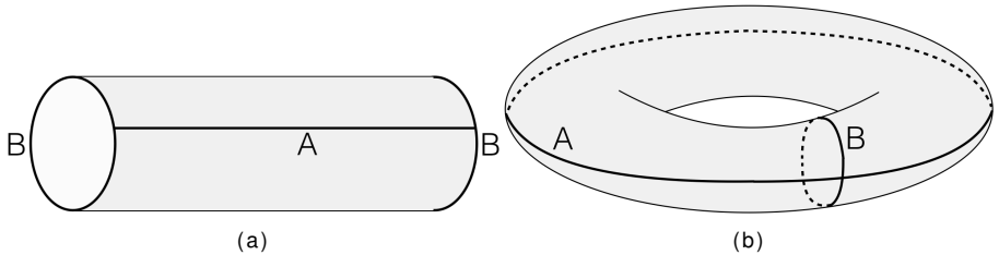
Abbildung 6: Zusammenkleben des Torus.
