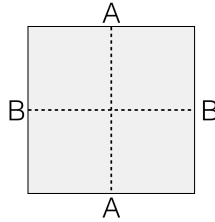
Abbildung 5: Identifizierung der Kanten eines Quadrates.
