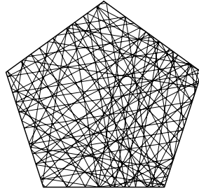
Abbildung 3: Eine Trajektorie auf einem fünfeckigen Tisch.
