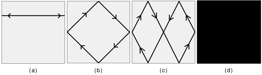
Abbildung 1: Unterschiedliche Pfade auf einem quadratischen Billardtisch.
