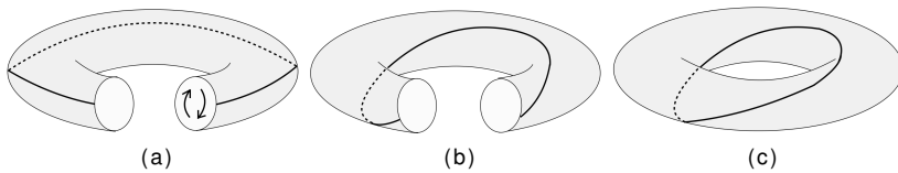
Abbildung 8: Der Torus wird durchgeschnitten, verdreht, und wieder zusammengeklebt.
