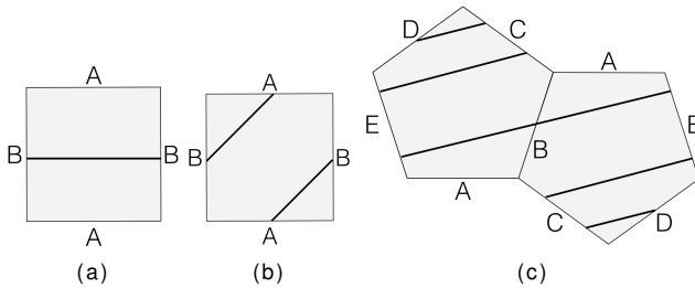
Abbildung 9: Die Verdrehung der Trajektorie auf einem Quadrat (a)-(b) und eine Trajektorie auf zwei Fünfecken (c).
